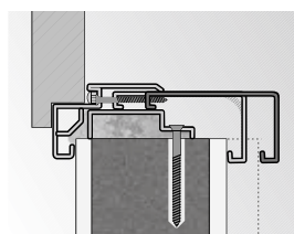
ościeżnica Regulowana
