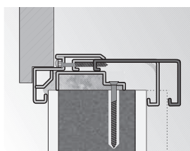
ościeżnica Regulowana
