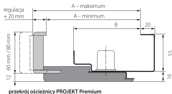
ościeżnica PROJEKT Premium
