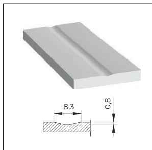
zbliżenie na frezowanie model 1
