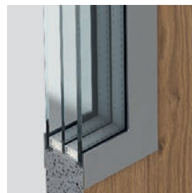
Przeszklenie – zestaw trzyszybowy klasa P4
