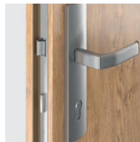
Zamek listwowy SAFE typ III, ENER- GY PROTECT
