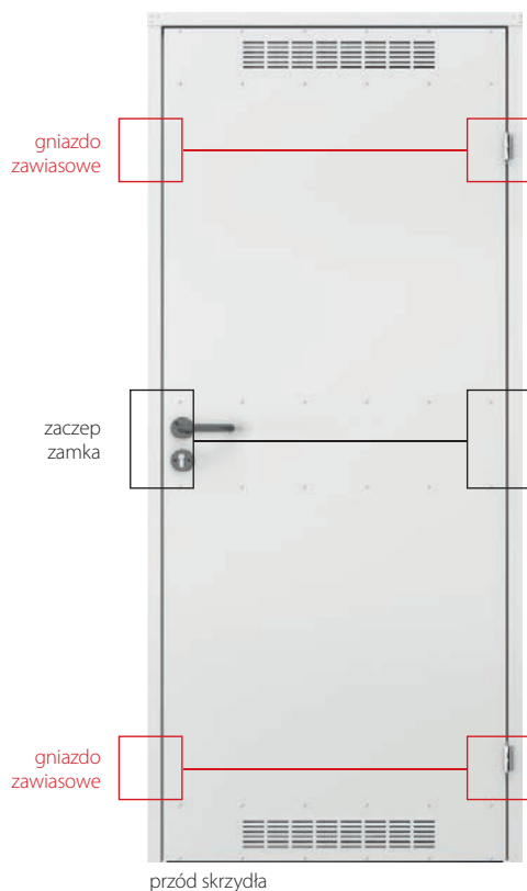
przód skrzydła
