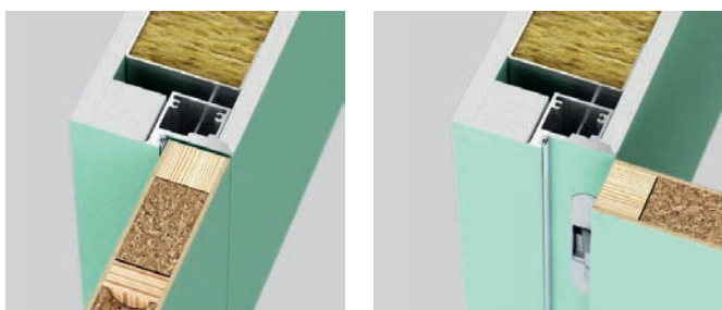
Bezprzylgowe standard (otwierane na zewnątrz) - drzwi prawe
