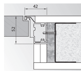
odwrotna przylga (otwierane do wewnątrz)
