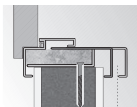
ościeżnica Regulowana „na kant”
